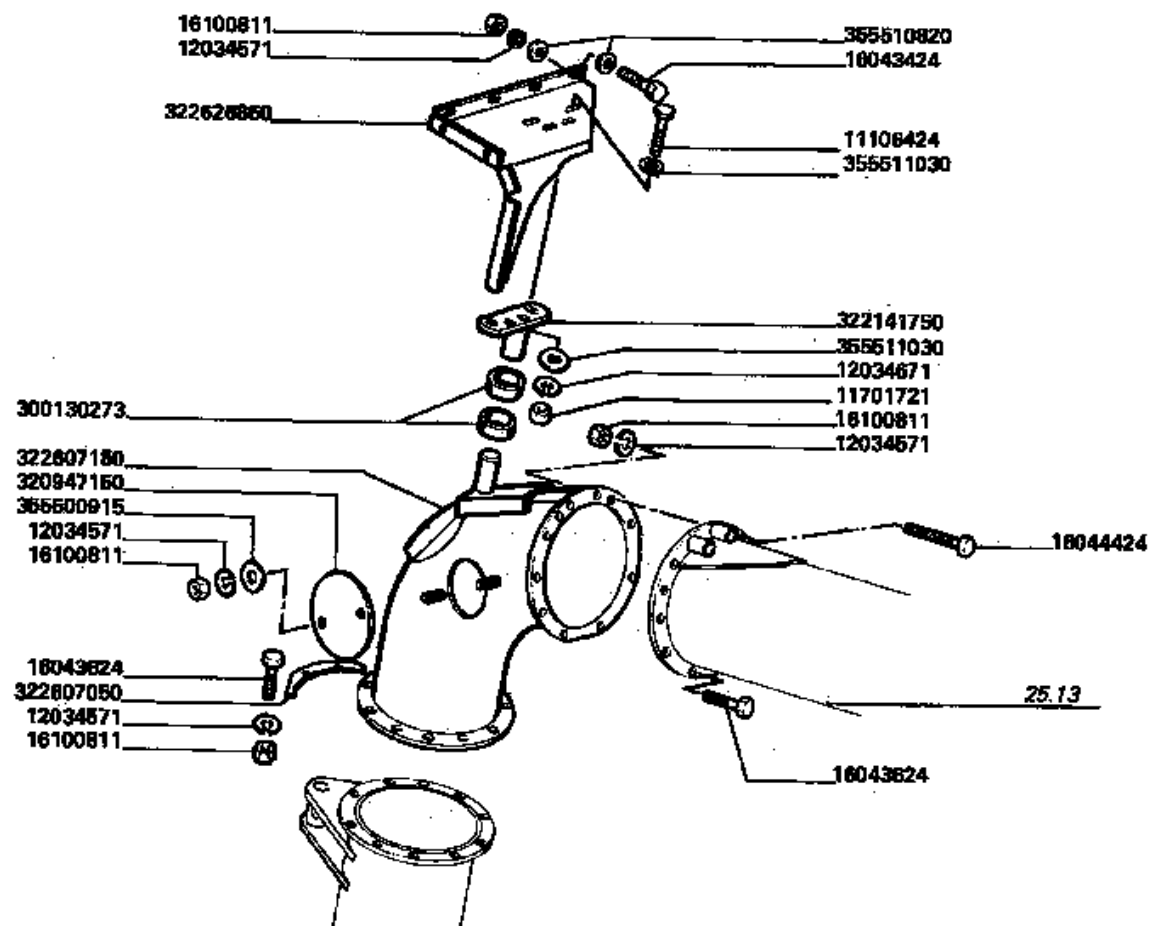
TUBO VERTICALE SCARICO SERBATOIO
