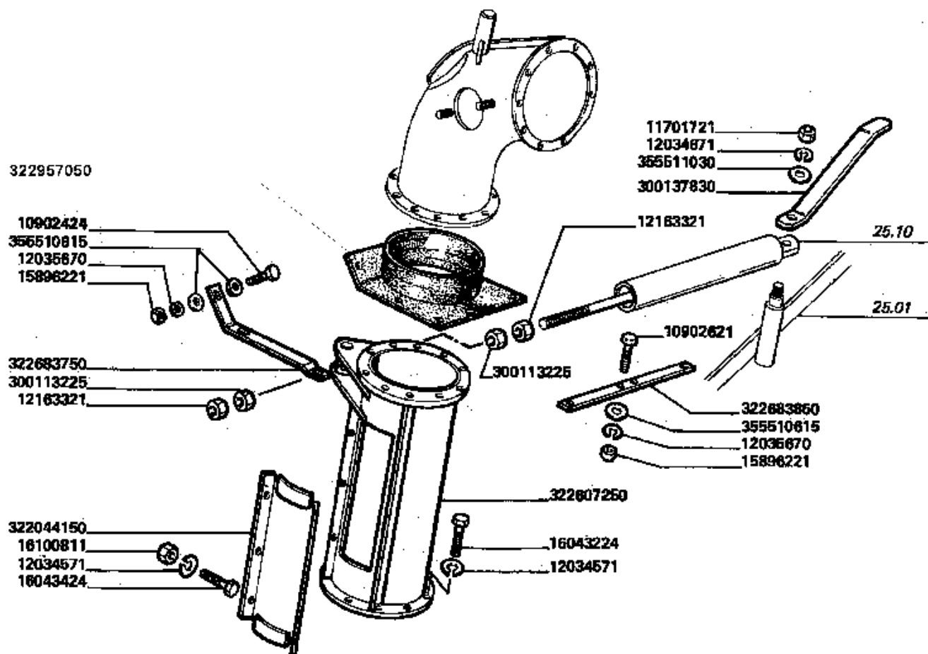
TUBO VERTICALE SCARICO SERBATOIO
